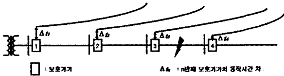
그림 5 보호기기 간의 보호협조 방식 Fig. 5 Protection and cooperation method among protective equipments
