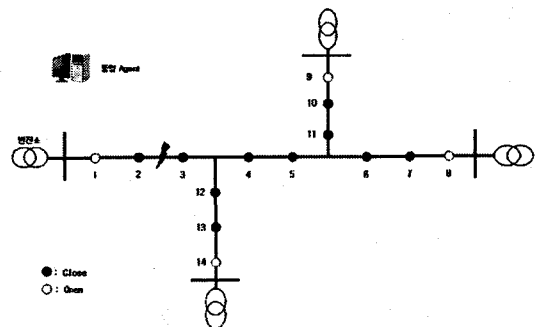
그림 7 예제 배전계통 Fig. 7 Four feeders example distribution system
