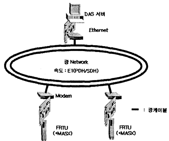
그림 4 이더넷 적용을 위한 MASX의 적용 구조 Fig. 4 Network structure for applying Ethernet
