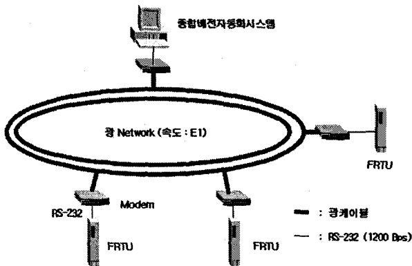
그림 2 국내 광전송로 기반의 배전자동화 통신망 구성 Fig. 2 Communication structure of Korean DAS
