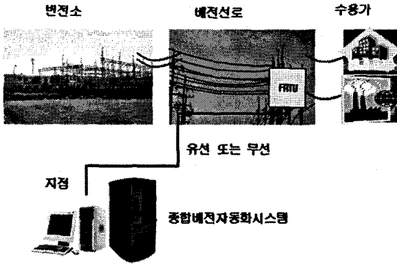
그림 1 배전자동화 시스템의 기본 구성 Fig. 1 General structure of distribution automation system
